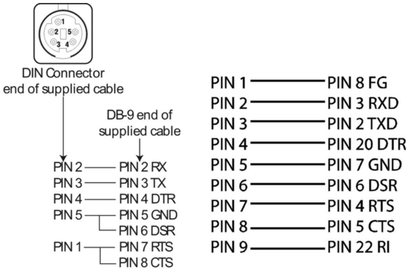
DIN to DB-9 Cable
